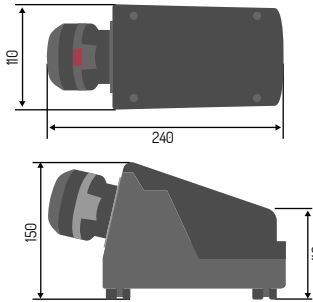
TOMADA/PLUG 16A
