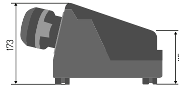
TOMADA/PLUG 32A
